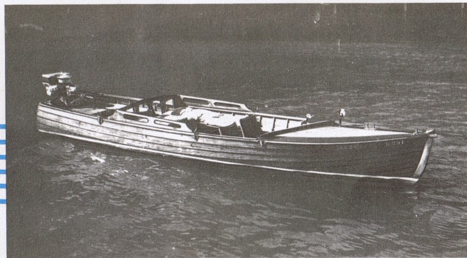
Familien-Aussenbord-Motorboot; Mahagoni; Länge 5,5 m; 8 Personen; Motor bis 12 PS.
